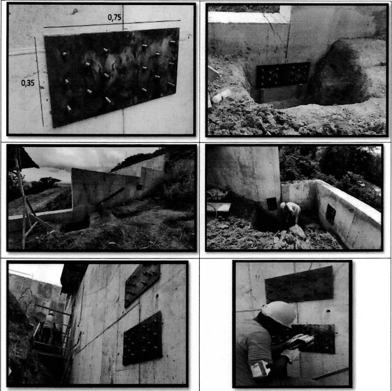
SUMINISTRO E INSTALACION DE PLANCHAS DE ACERO ESTRUCTURAL COMO REFORZAMIENTO AL MURO
