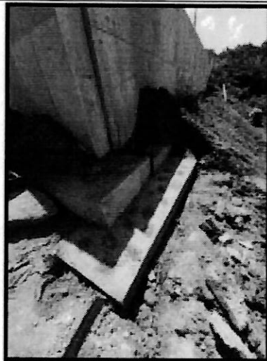
CONCRETO CICLOPEO COMO BASE DE CIMENTACION MURO FRONTAL CON SU RESPECTIVO DISIPADOR
