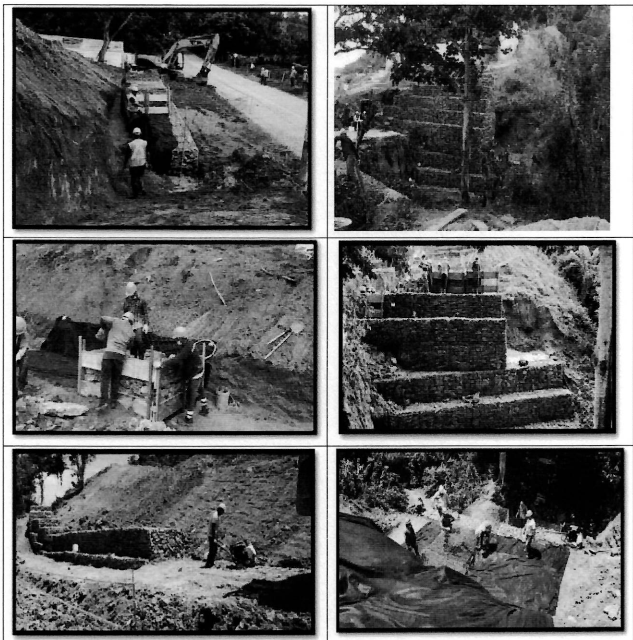
COLOCACION DE GAVIONES INCLUYE EL LLENADO LA PIEDRA PARA GAVION Y EL GEOTEXTIL
