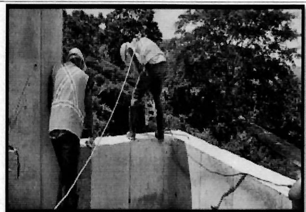
COLOCACION VARILLA TENSORAS
